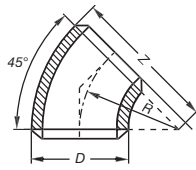
Rohrbogen Typ A, verminderter Ausnutzungsgrad
