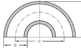
Rohrbogen 180°
