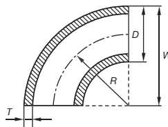
Rohrbogen 90°
