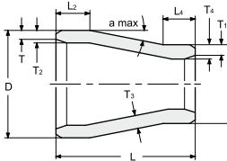
Konzentrische Reduzierung nach DIN EN 10253 Typ B
