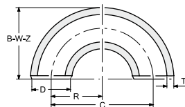
Rohrbogen nach DIN EN 10253 Typ A
